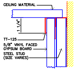
2 PANEL ON STUD
